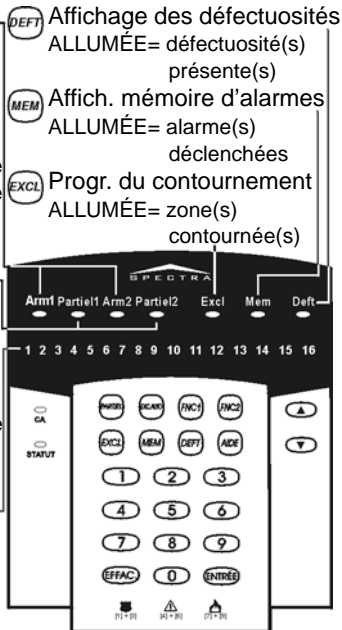
Figure 2 : Vue d'ensemble du clavier à DEL 1689
